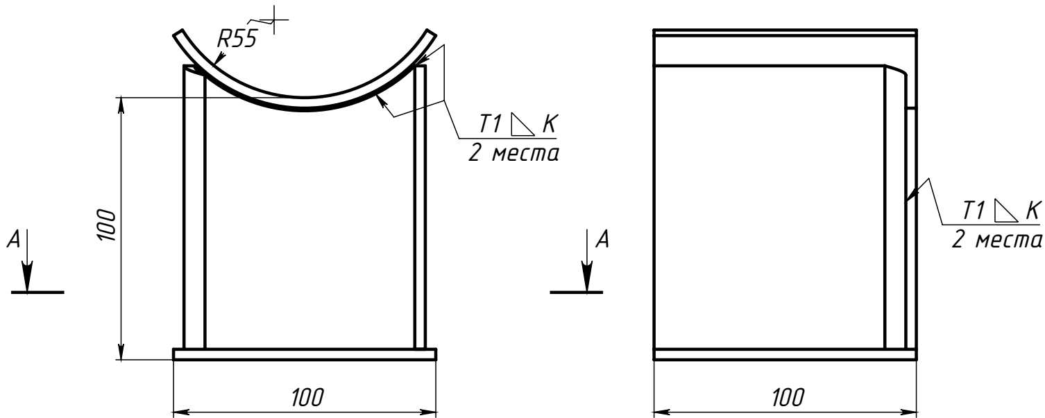
Поз.3 (Ложемент)
