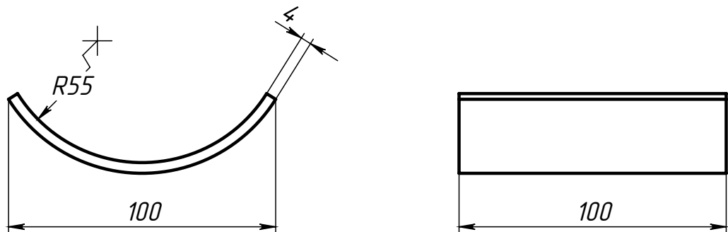
Поз.3 (Ложемент)
