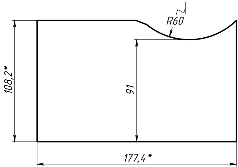
Поз.2 (Угольник)
